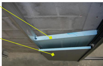
Plan en coupe (vue de dessus)
